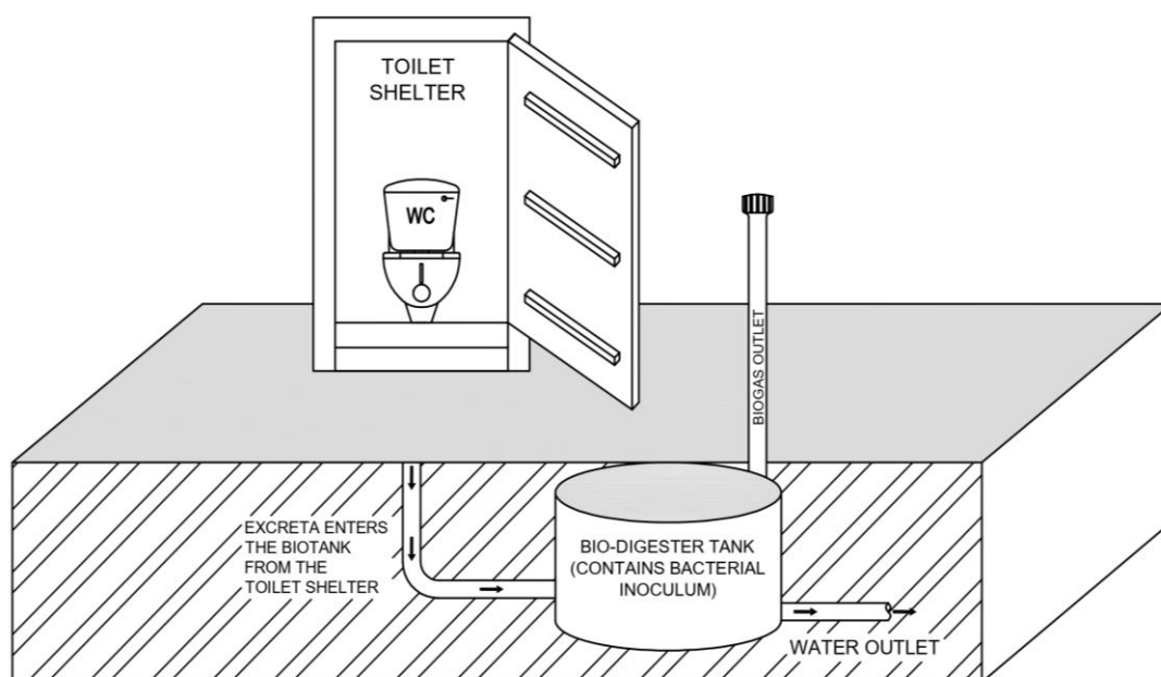
Fig. 5 BIO-TOILET (OR ECO-TOILET)
