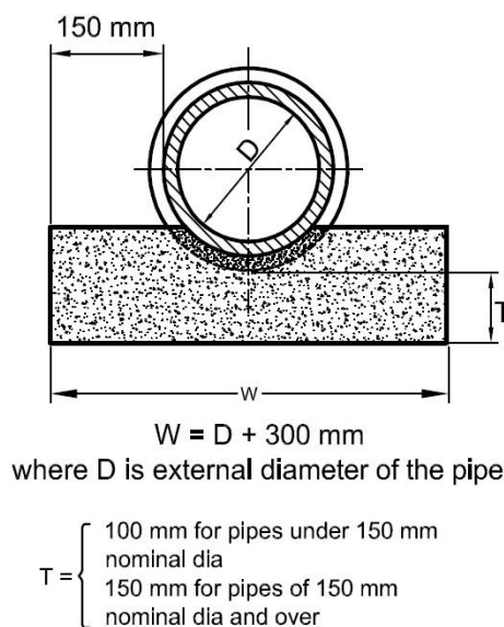
FIG. 15 BEDDING
