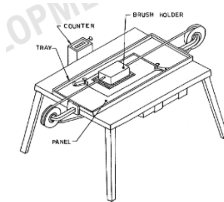
FIG. 1 WET ABRASION TESTER
