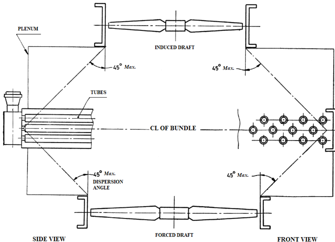
FIG. 8 FAN DISPERSION ANGLE
